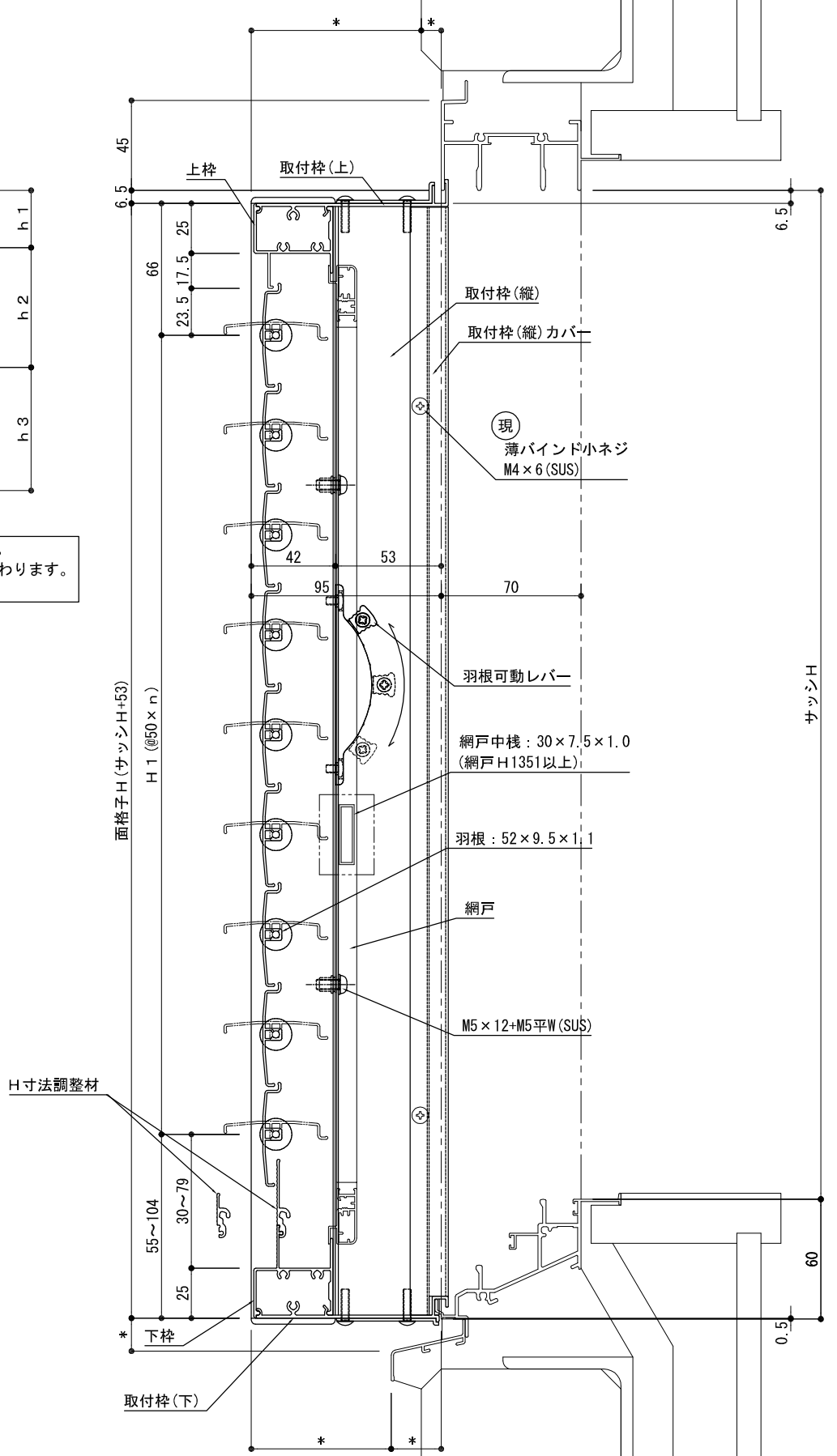
断面詳細図
