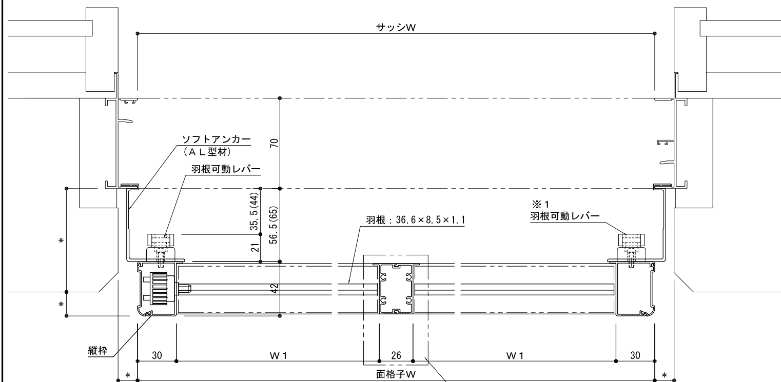
平面詳細図
