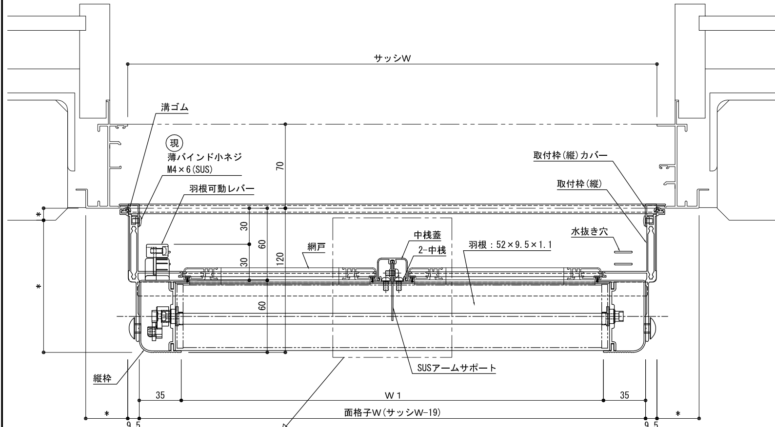
平面詳細図
