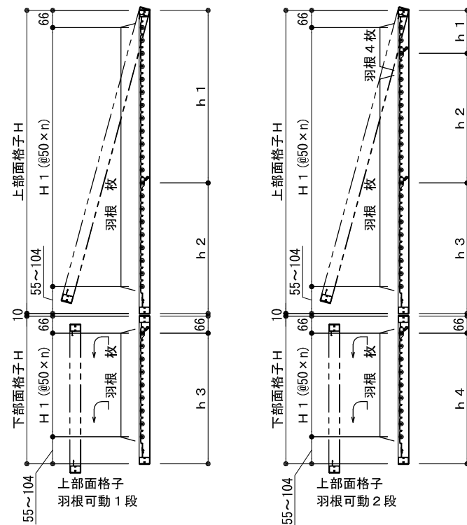
シングル(アームサポートなし) ダブル(アームサポートあり) 外観姿図
