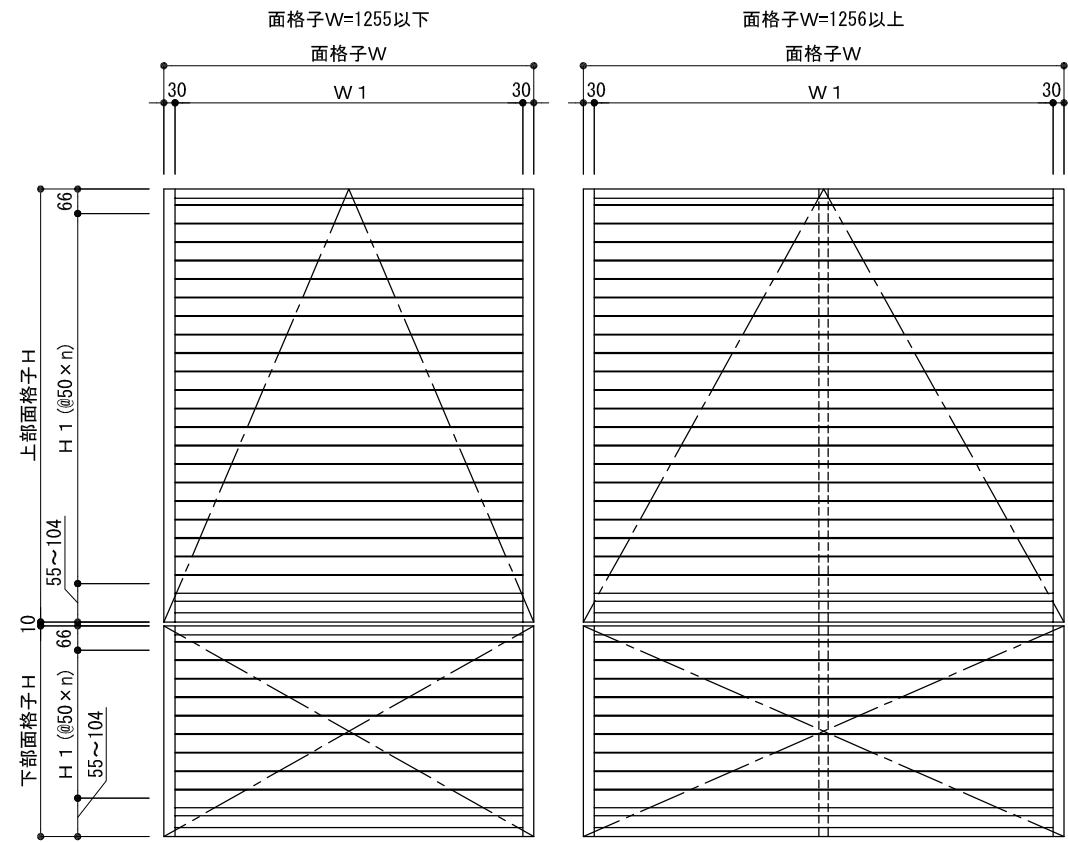
シングル(アームサポートなし) 外観姿図 ダブル(アームサポートあり)
