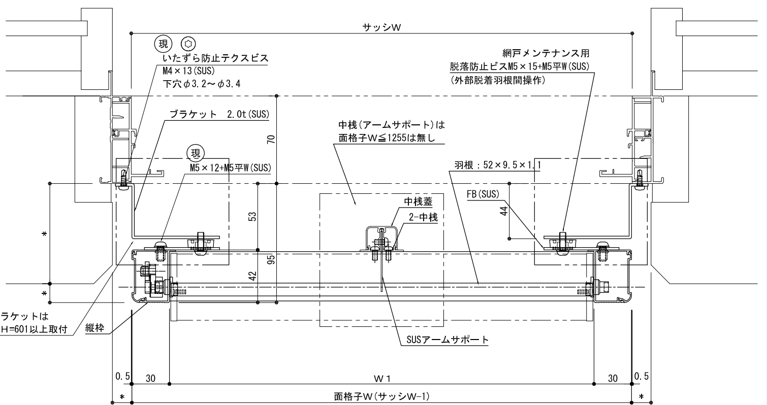
下部FIXサッシ部 平面詳細図
