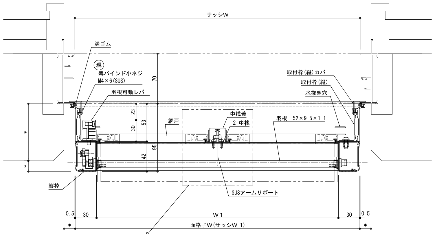
上部引違サッシ部 平面詳細図
