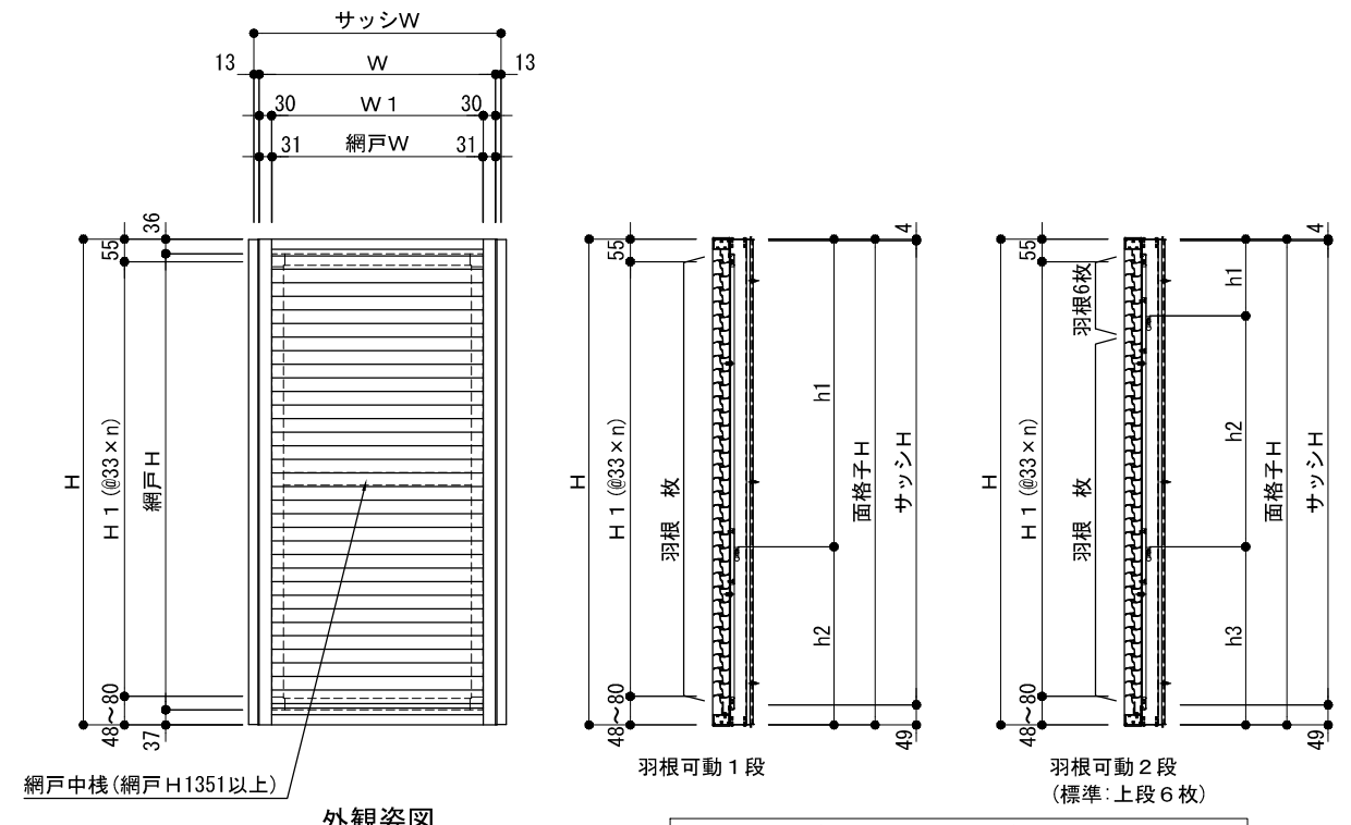
外観姿図
