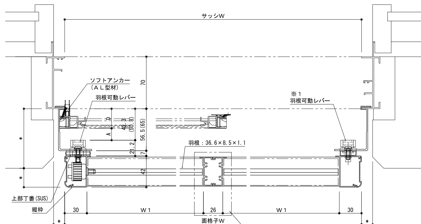
平面詳細図
