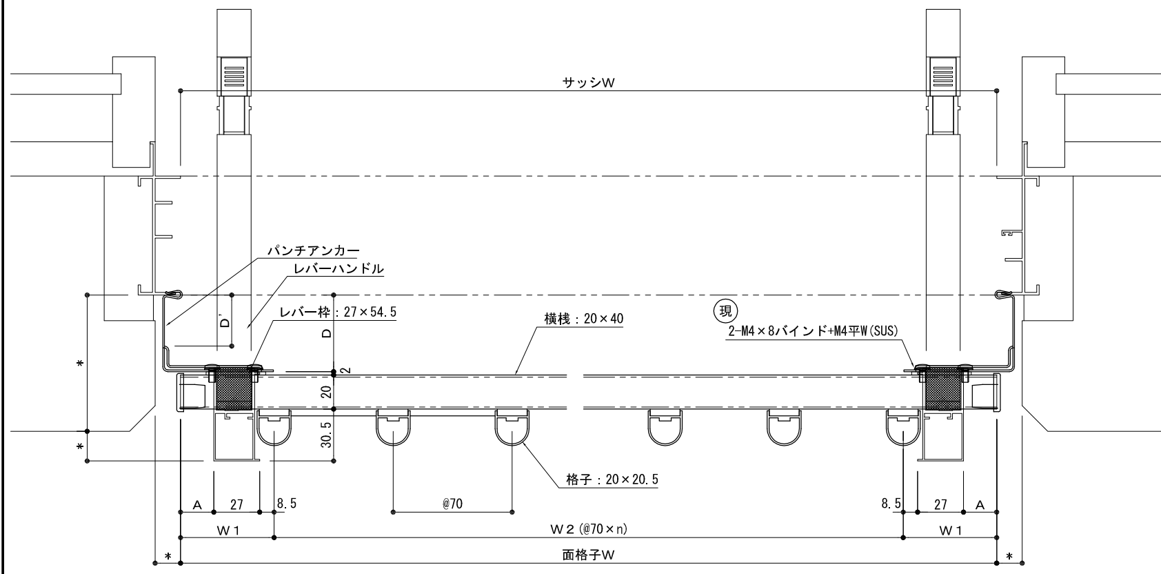
平面詳細図
