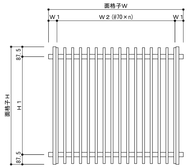
外観姿図
