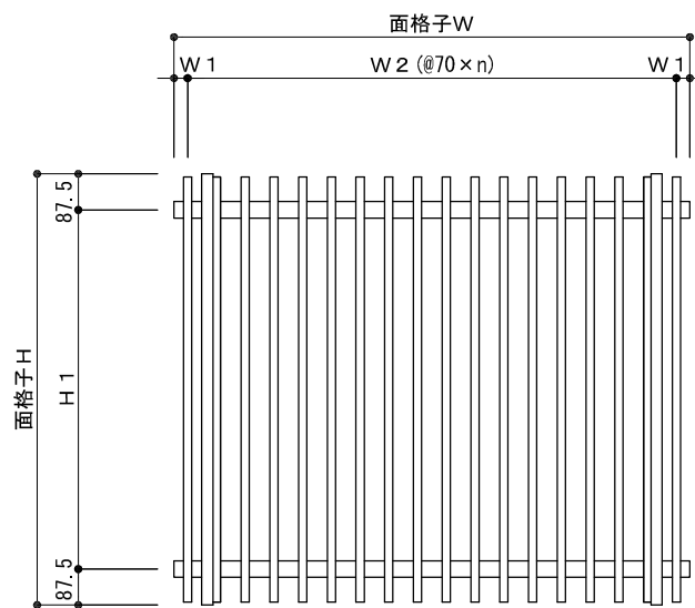
外観姿図
