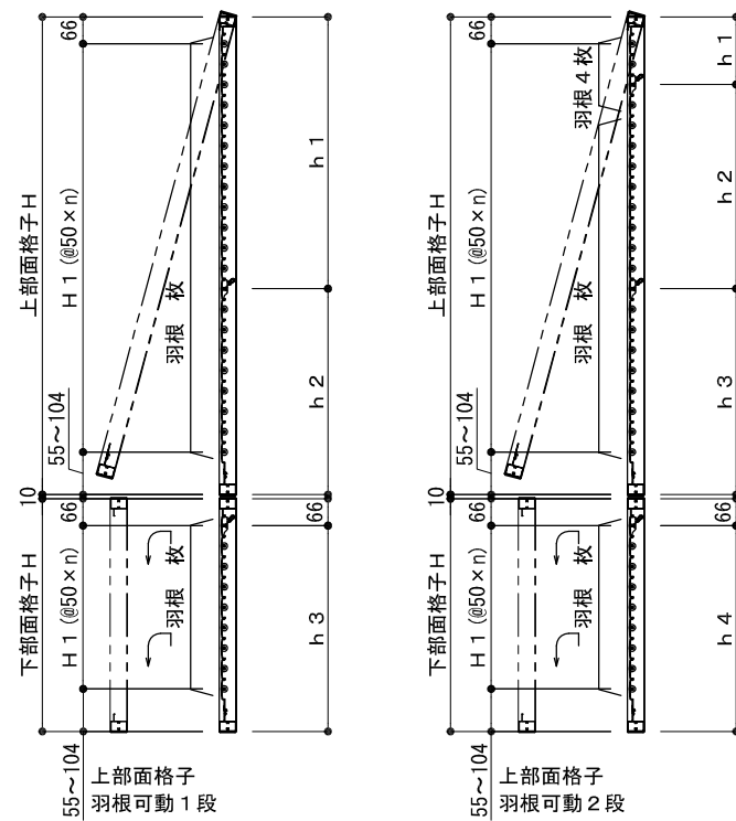
外観姿図
