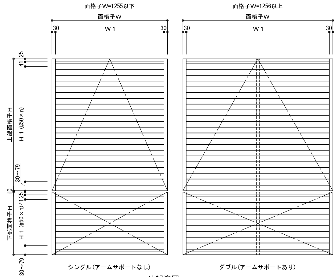
外観姿図
