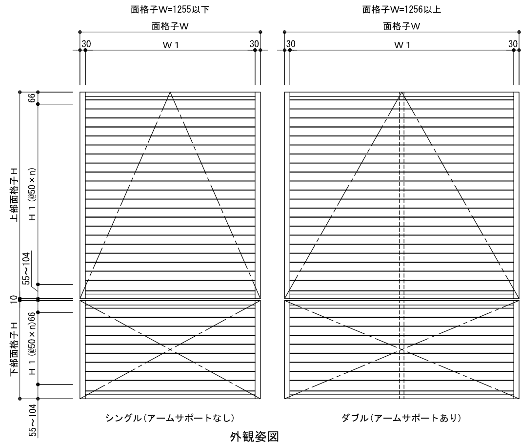
外観姿図
