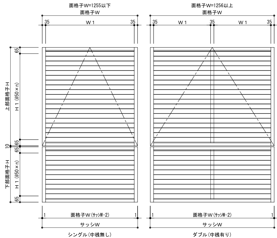
外観姿図
